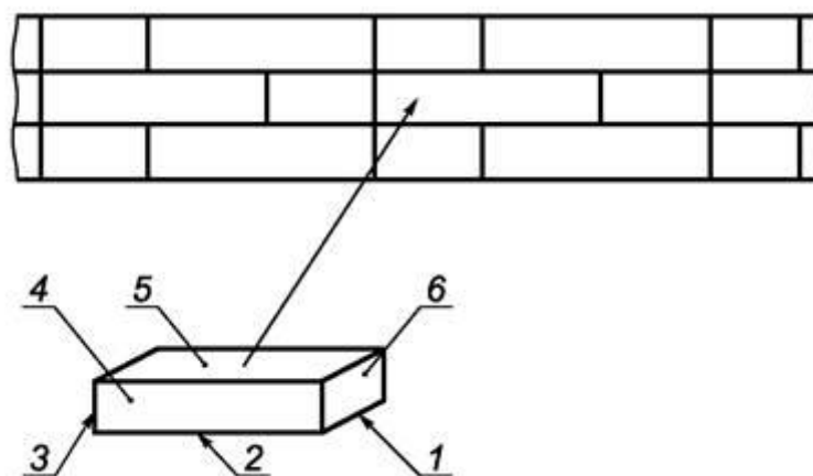
Рисунок 1 - Фрагмент кладки 2
